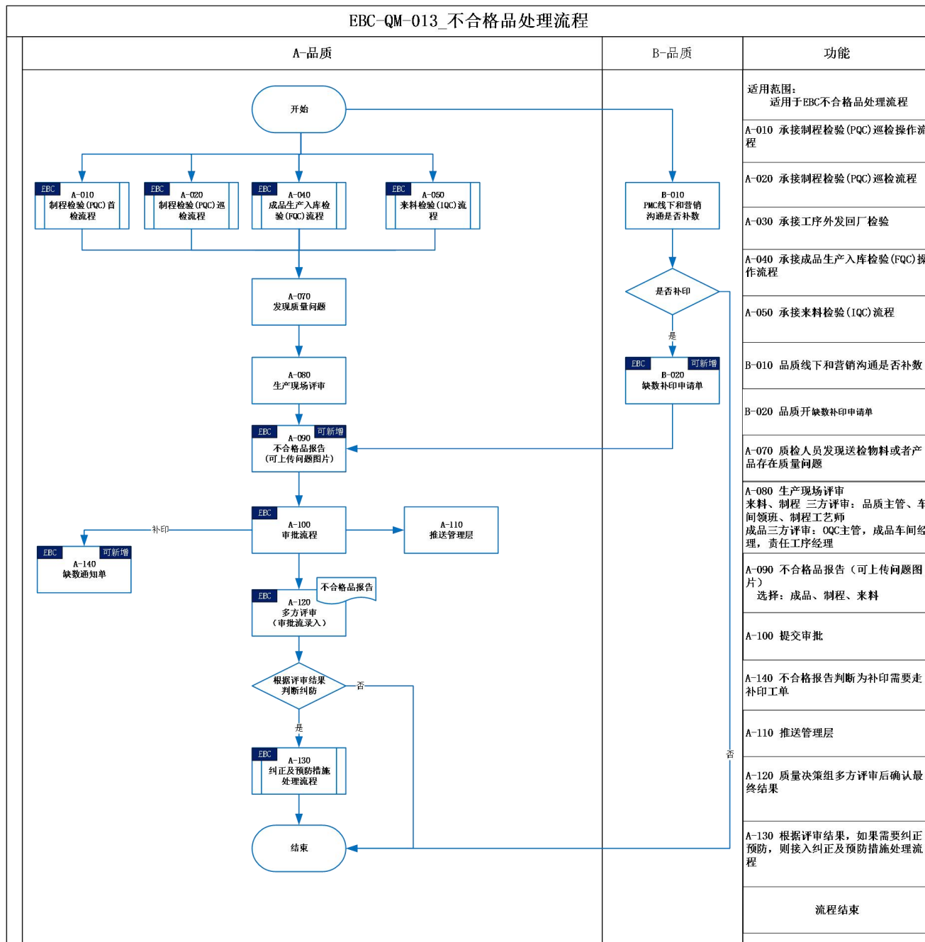
图 2 流程图
