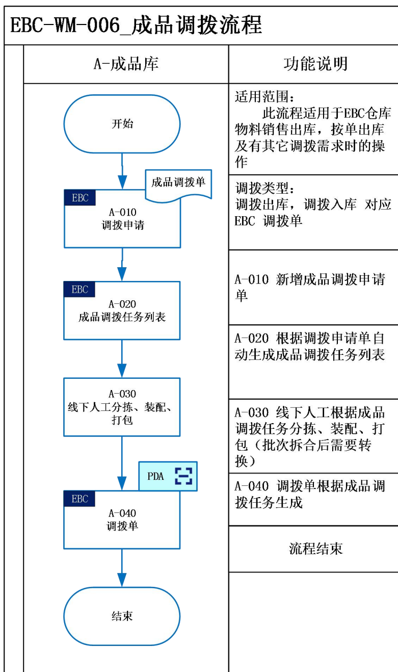
图 2 流程图
